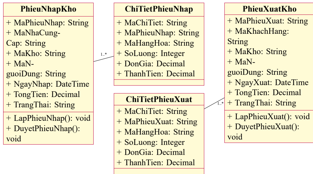
Hình 1: Sơ đồ lớp nghiệp vụ nhập xuất kho
